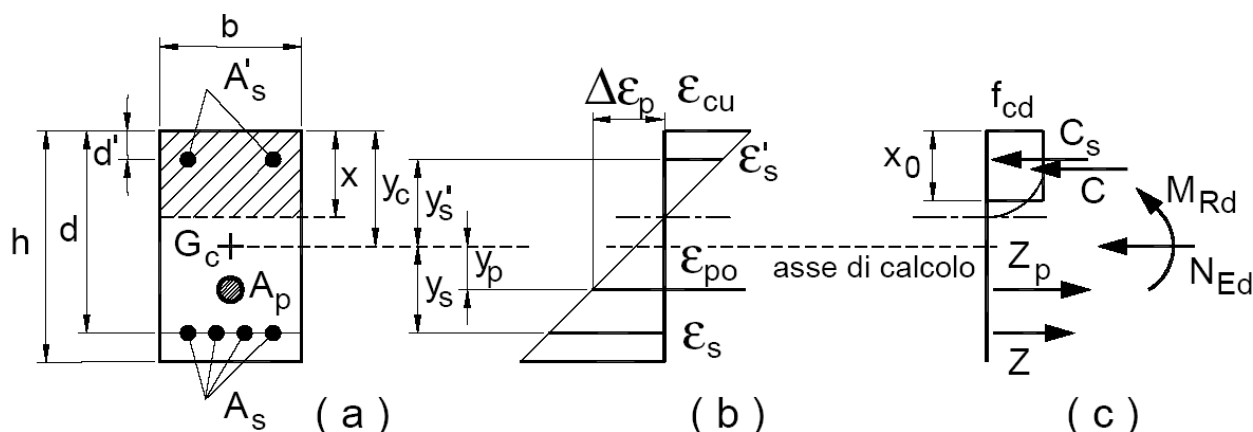
Figura 4.1.3– Sezione pressoinflessa
